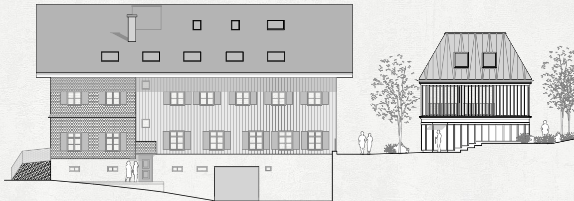
ANSICHT NORD 1:1300
