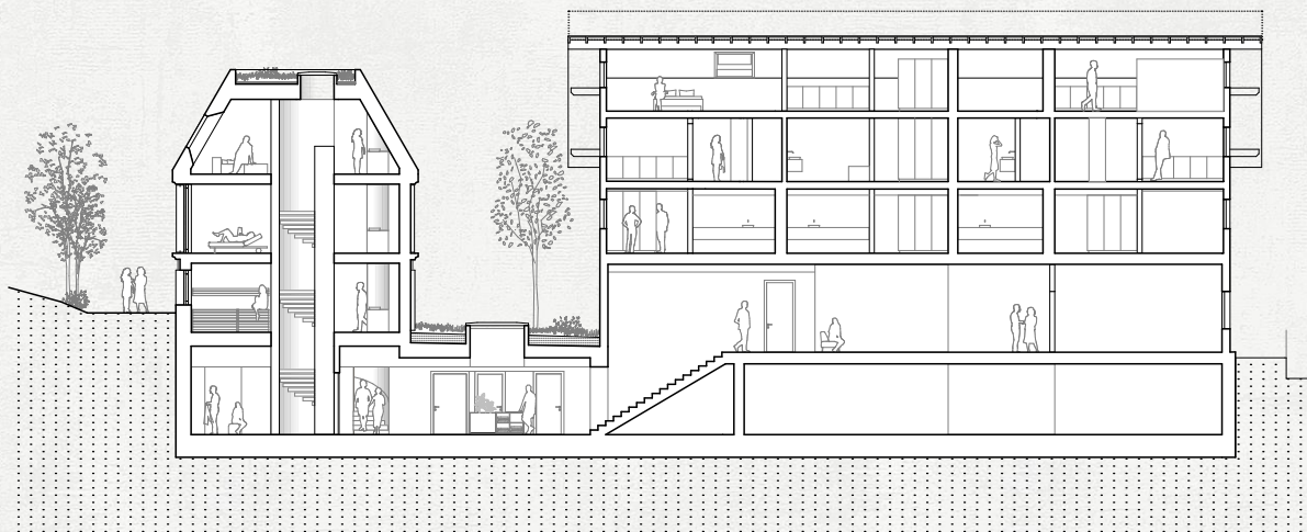
SCHNITT 1:1300
