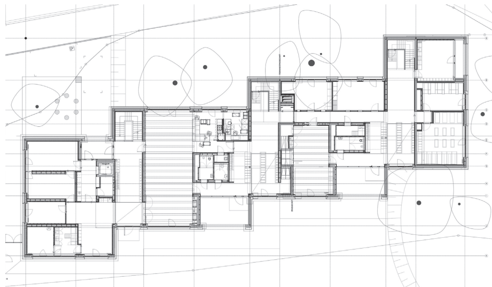
EG
