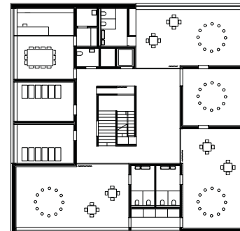
Obergeschoss Kinder, Verwaltung, Schlafen, Atelier
