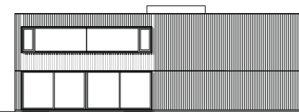
Ansicht Nord
