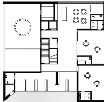
Erdgeschoss Gartenspiele, Kleinkinder, Essen, Bewegung
