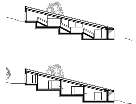
Längsschnitt
